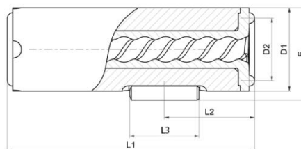
D1 = Ø 11,95 mm L1 = 35,50 mm L3 = 10,00 mm D2 = Ø 9,00 mm L2 = 13,00 mm E = 13,25 mm
